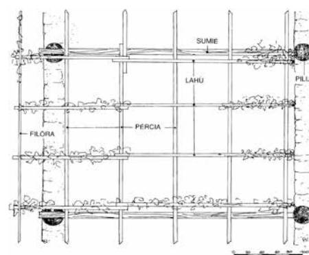
• Schema di un pergolato-Pianta
