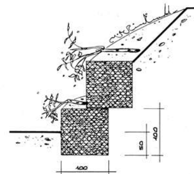
GABBIONATA CON TALEE
