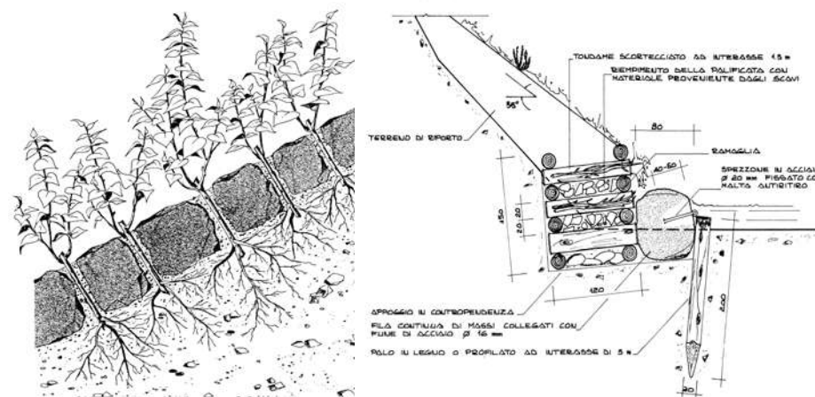
Sezione
