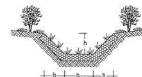
• Estratto Quaderno opere tipo Autorità di Bacino fiume Po.
