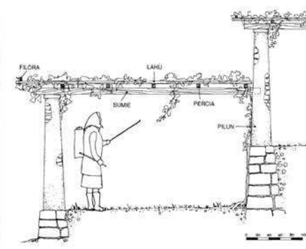
• Schema di un pergolato-Sezione
