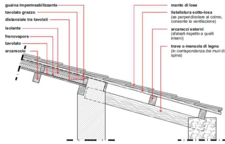
Figura 127: struttura ad arcarecci per copertura in lose ed isolante
