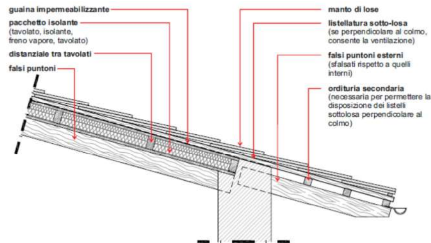
Figura 128: struttura a falsi puntoni con ventilazione sotto losa
