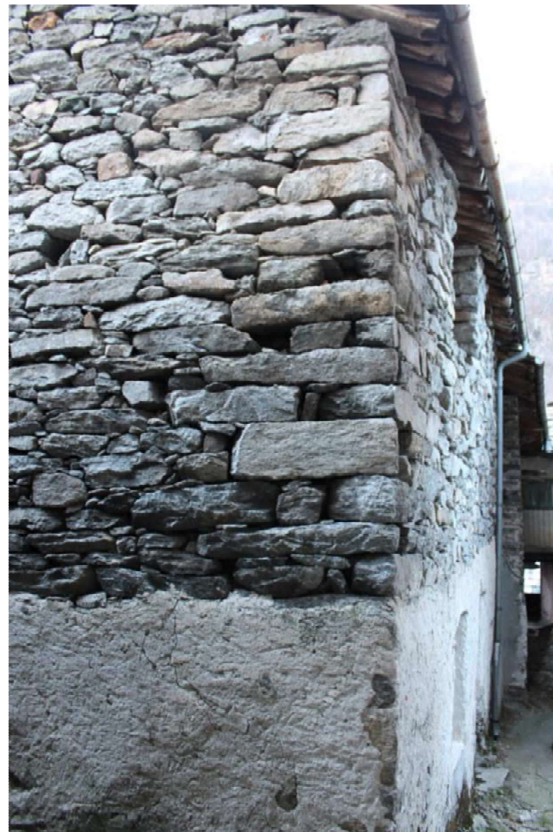
Figura 77: particolare dell'ammorsamento angolare
